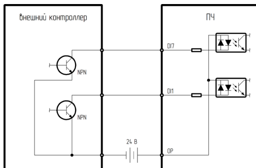
Рис. 3.12 - Режим подключения внешнего источника тока с логикой NPN
